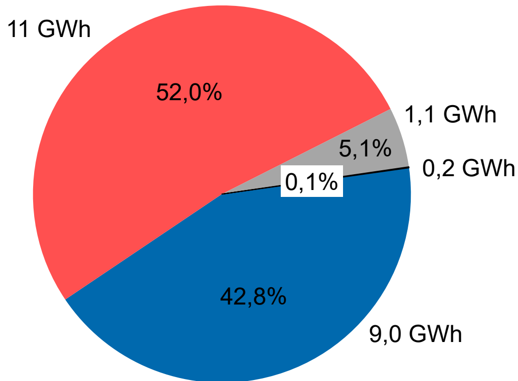
Energie-Bilanz 2023
